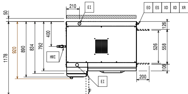
Felülnézet
